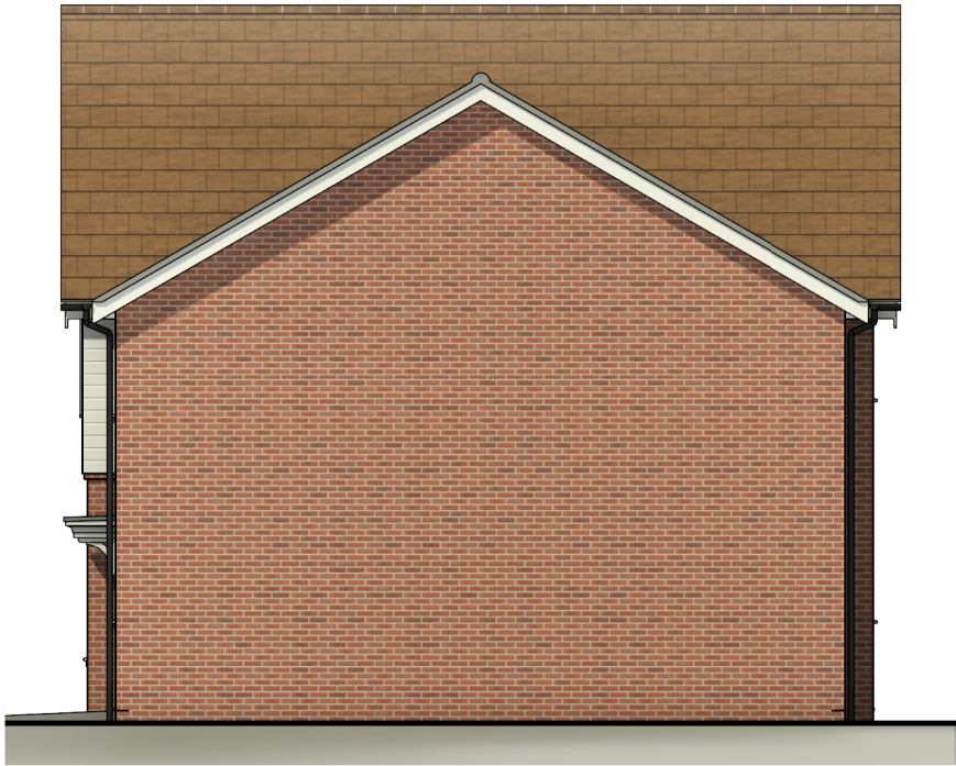
Right Elevation P065
