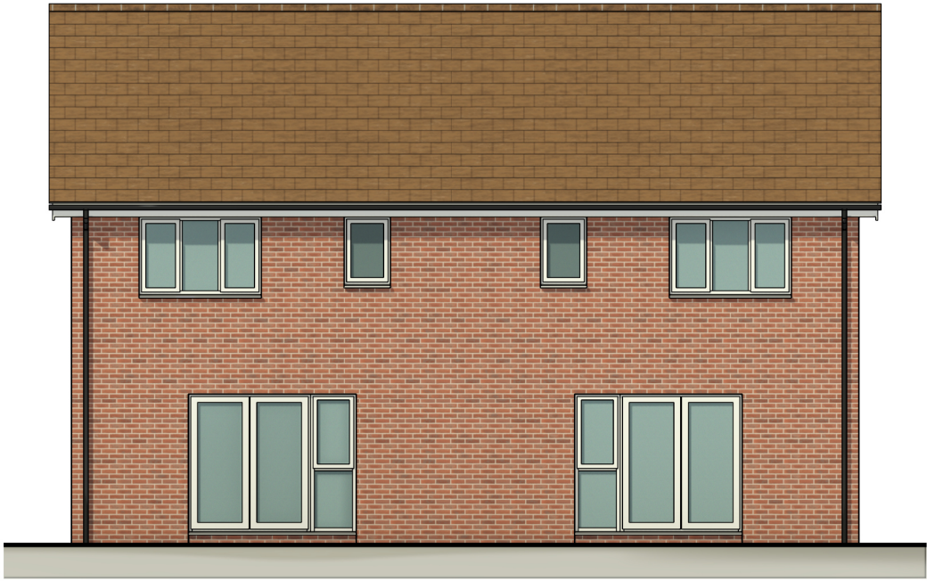
Rear Elevation P083 P082
