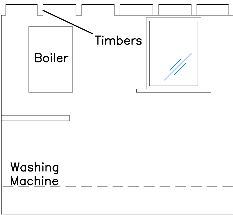
Elevation 6 1:20
