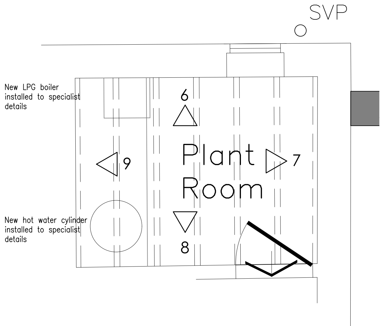
Plan 1:20
