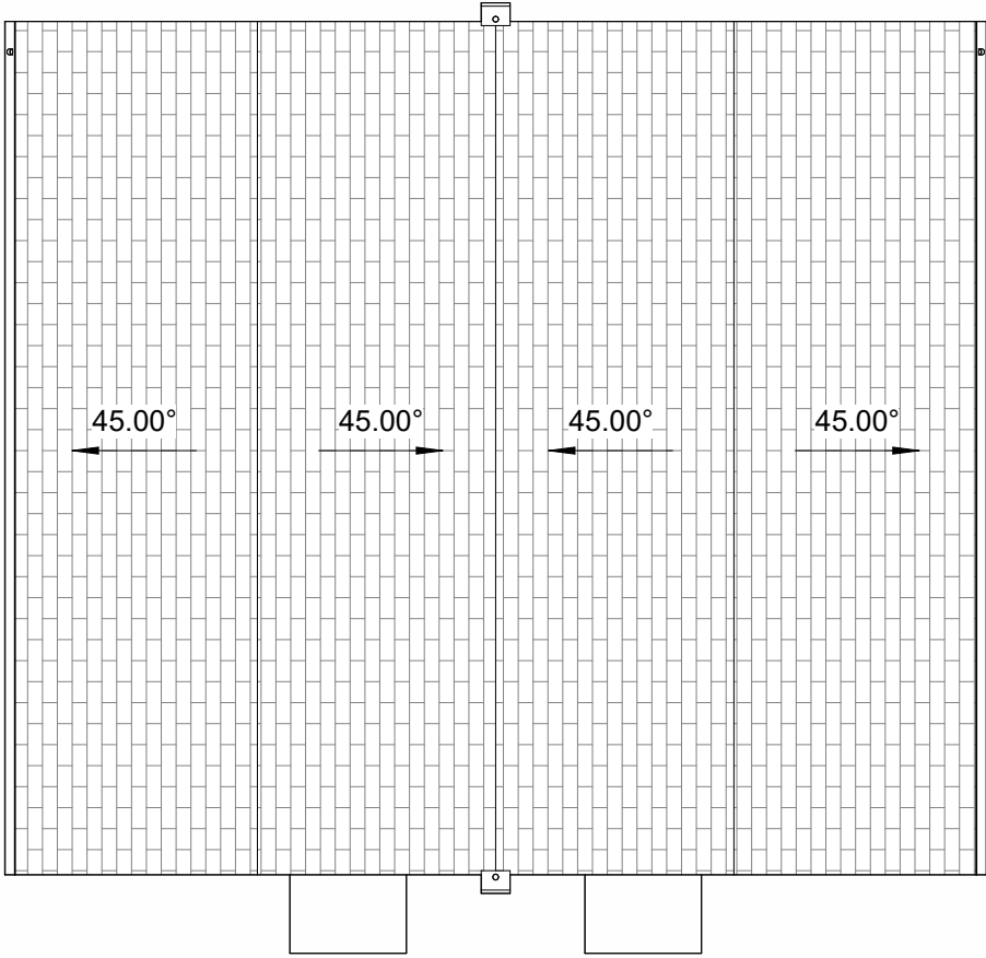
Roof Plan 1 : 100
