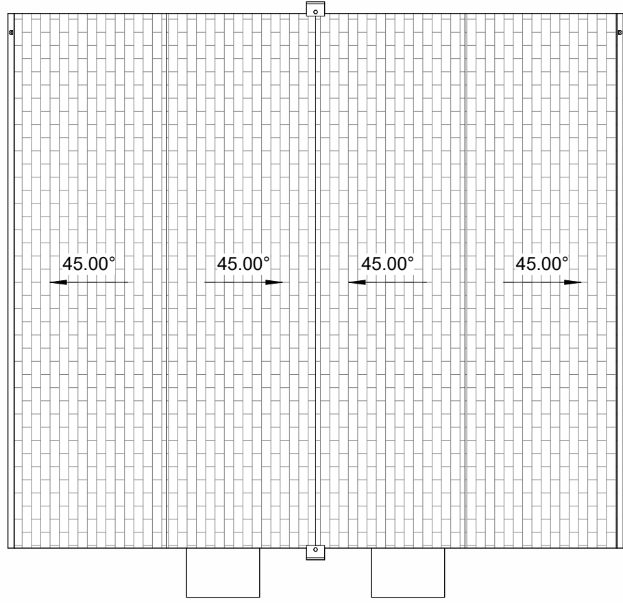
Roof Plan 1 : 100
