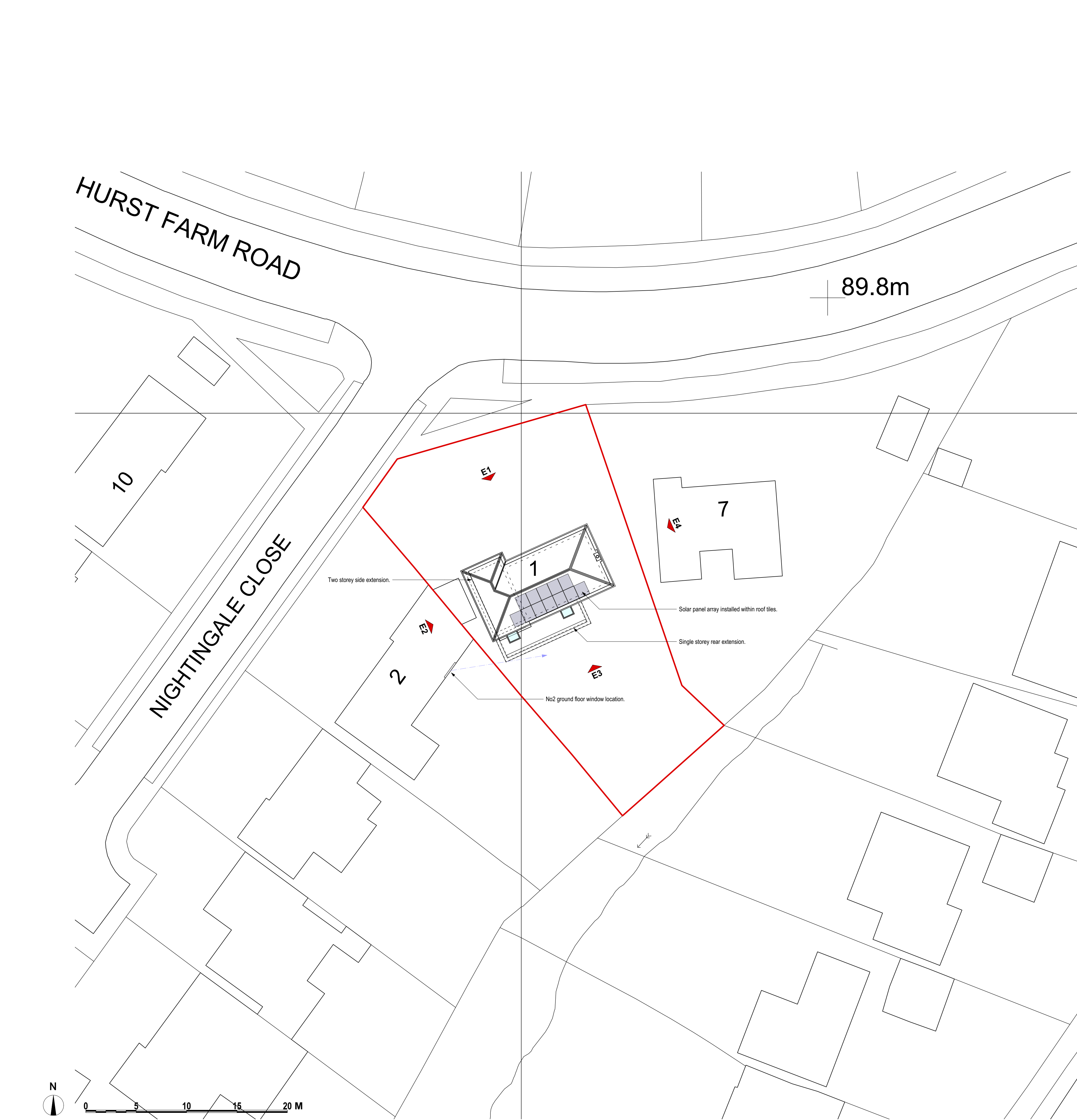
BP BLOCK PLAN Scale: 1:200
