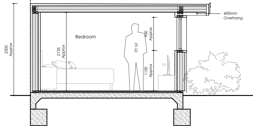
Section A-A Scale 1/50@A3
