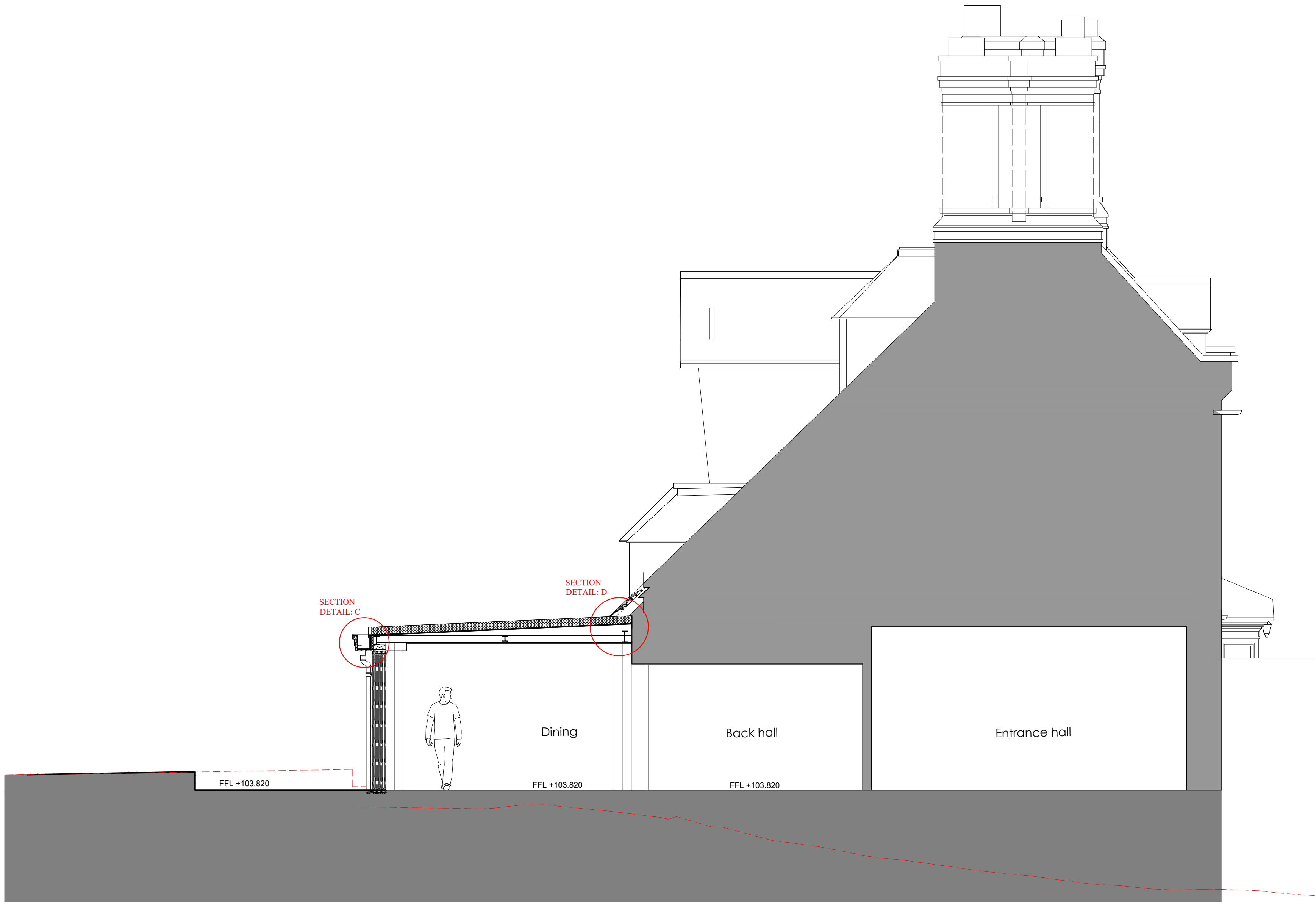
SECTION A-A
