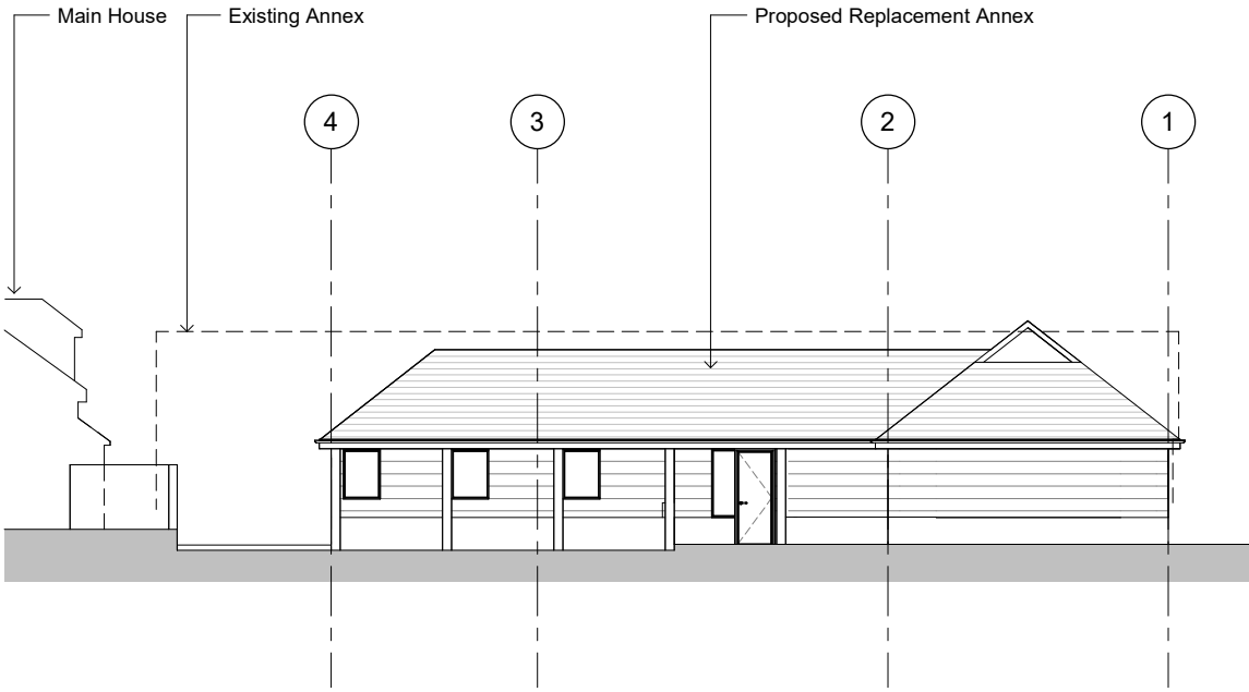
West 1 : 100
