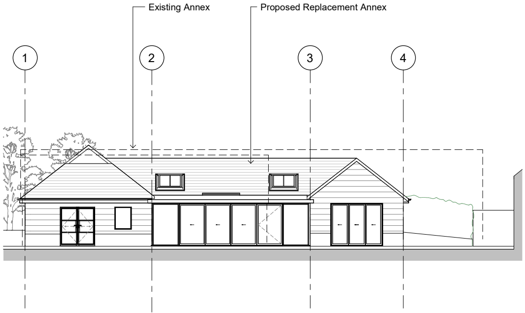
East 1 : 100
