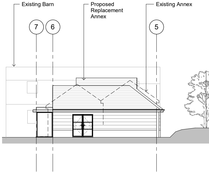
North 1 : 100
