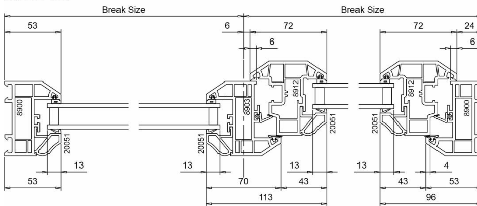
Section D-D
