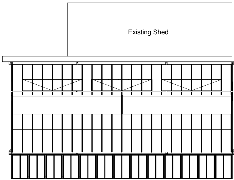
C Glasshouse - Plan Scale: 1:100
