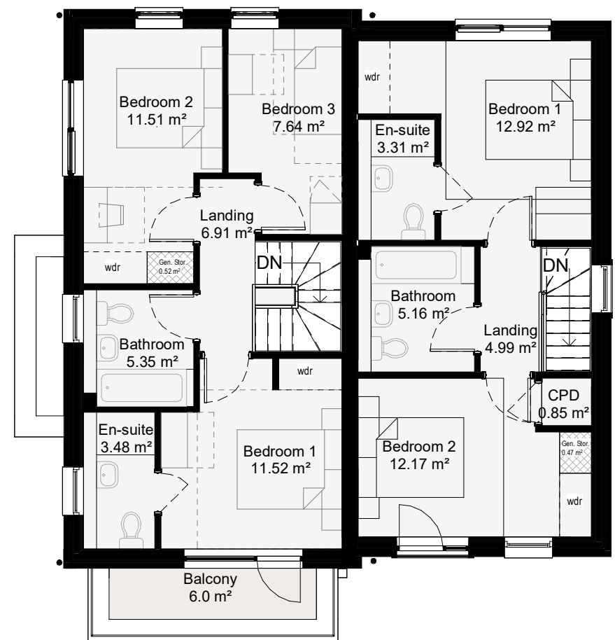
01 First FFL 1 : 100
