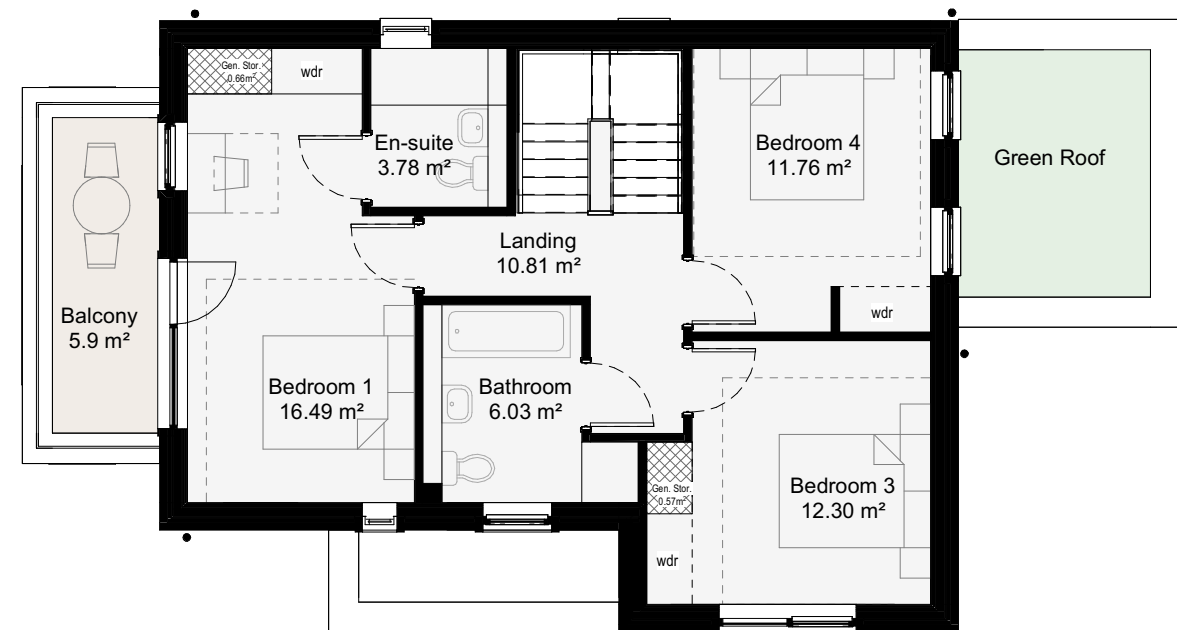
01 First FFL 1 : 100
