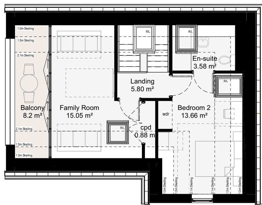
02 Second FFL 1 : 100
