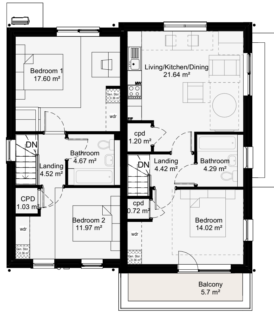
01 First FFL 1 : 100
