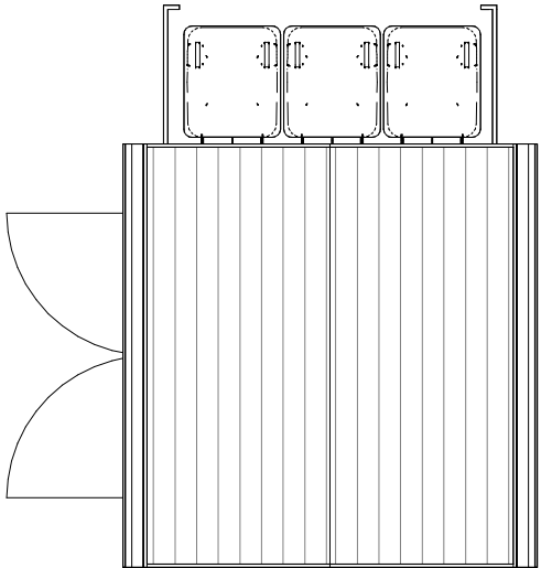
Roof Plan 1 : 50
