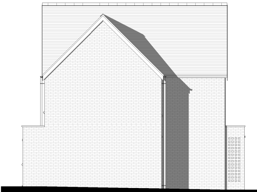
Left Flank Elevation
