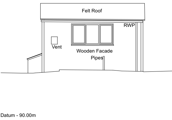
Elevation 17
