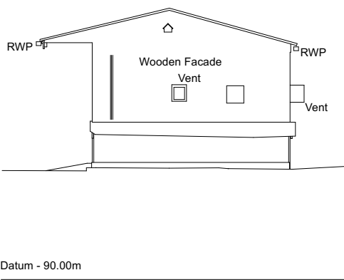
Elevation 16
