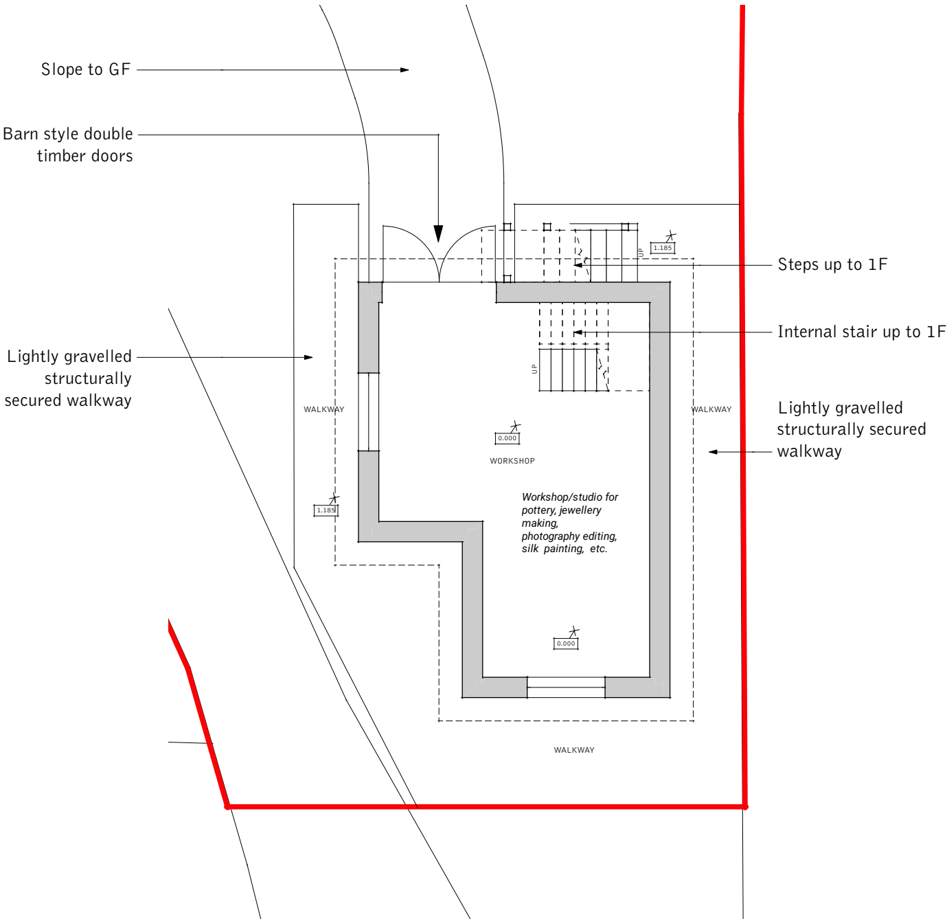
1 GF Plan Scale: 1:100 0 1 2 3 4 5 M
