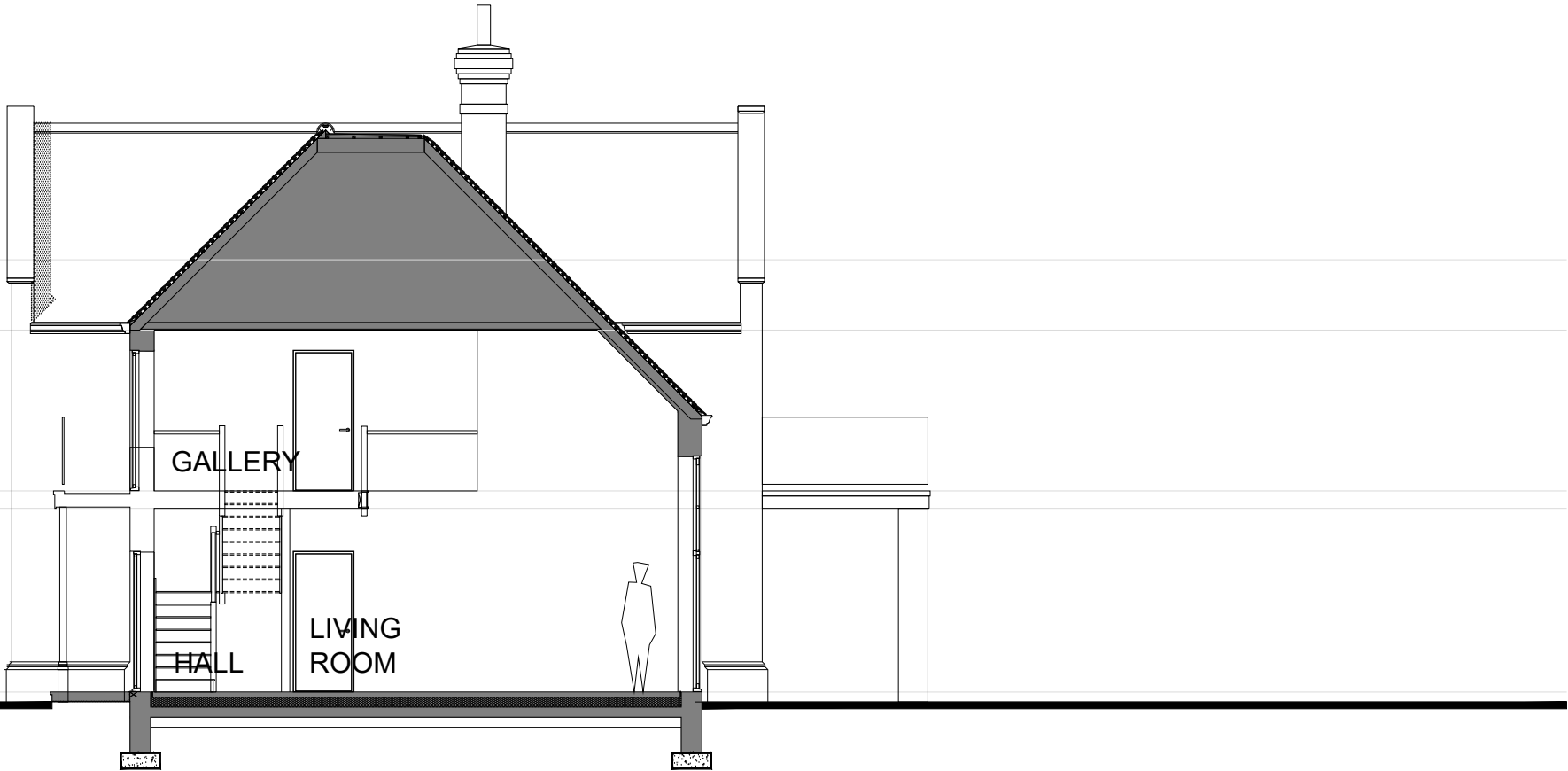
SECTION A-A
