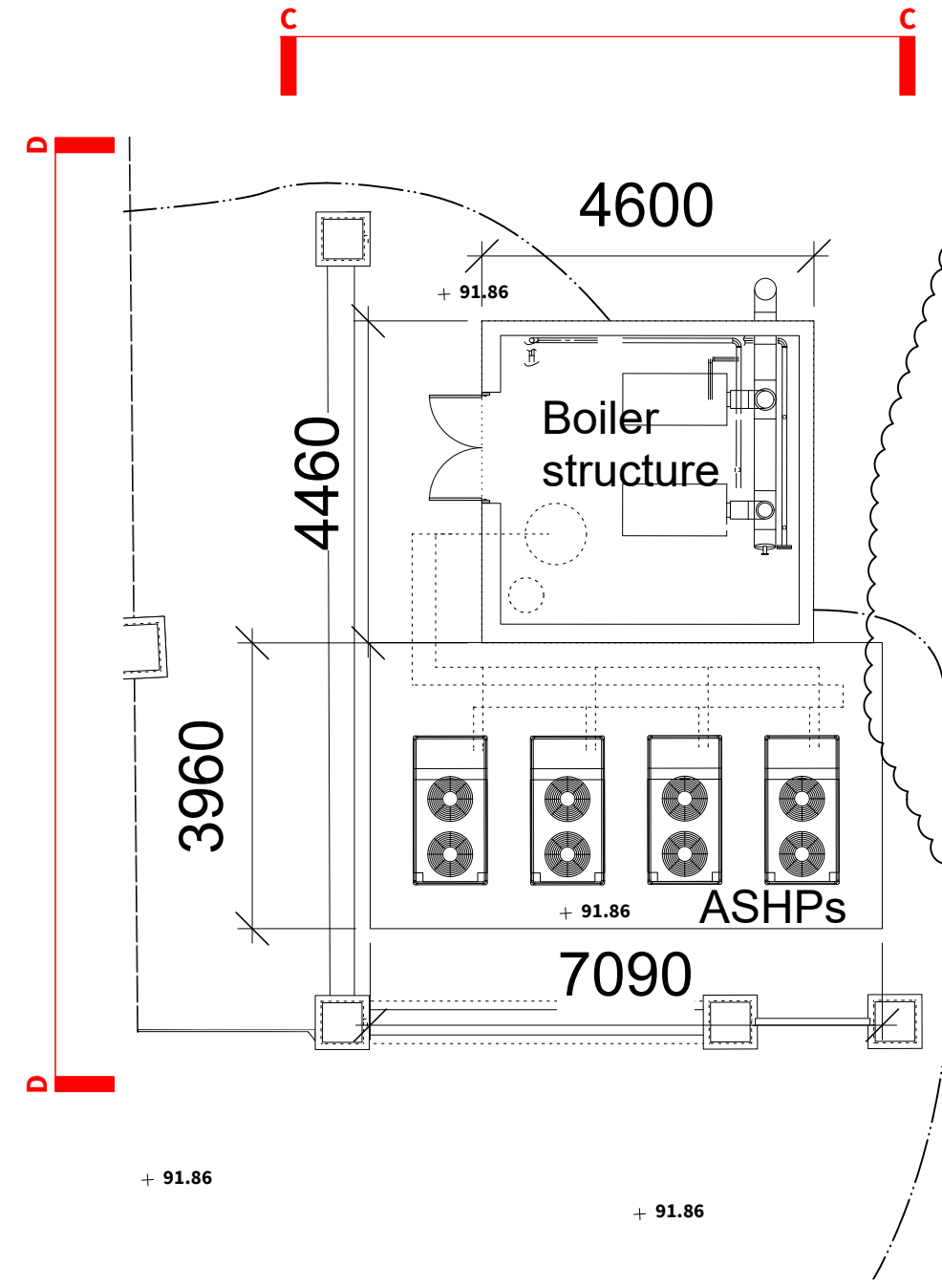
Key Plan 1:100 @A1
