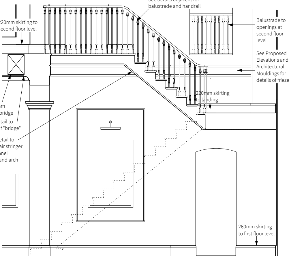
Section BB 1:50 @A3 / 1:25 @A1
