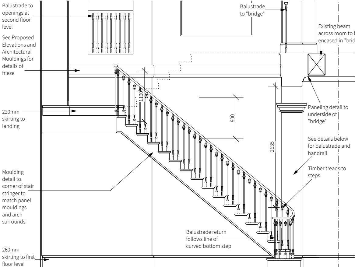
Section AA 1:50 @A3 / 1:25 @A1
