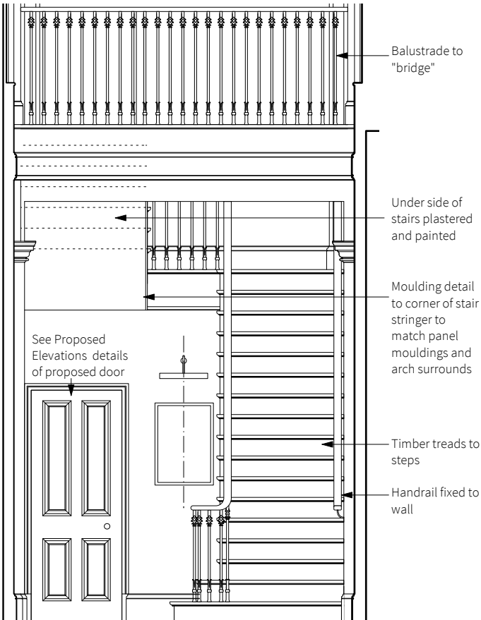
Section CC 1:50 @A3 / 1:25 @A1
