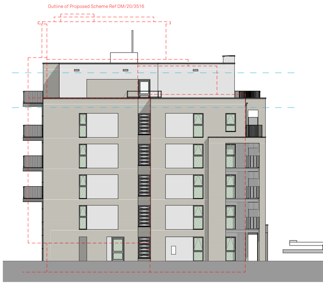
1:200 E-02 Elevation
