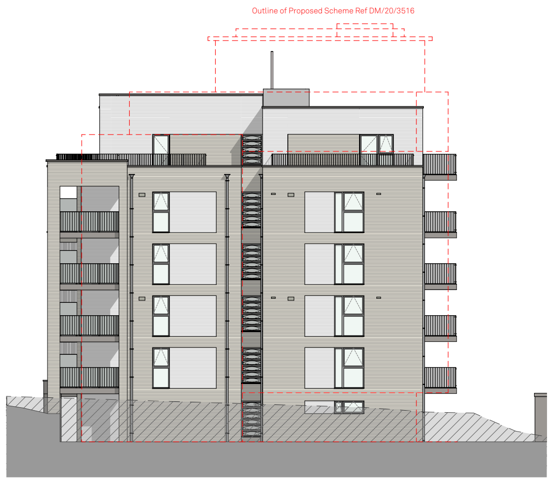
1:200 E-04 Elevation
