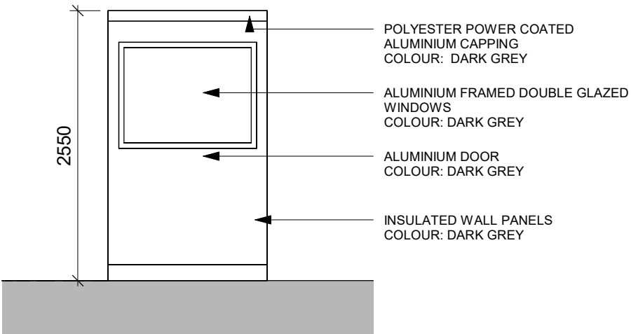
ELEVATION B 1:50
