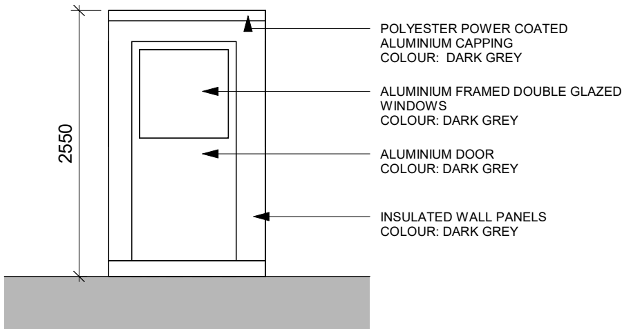
ELEVATION A 1:50
