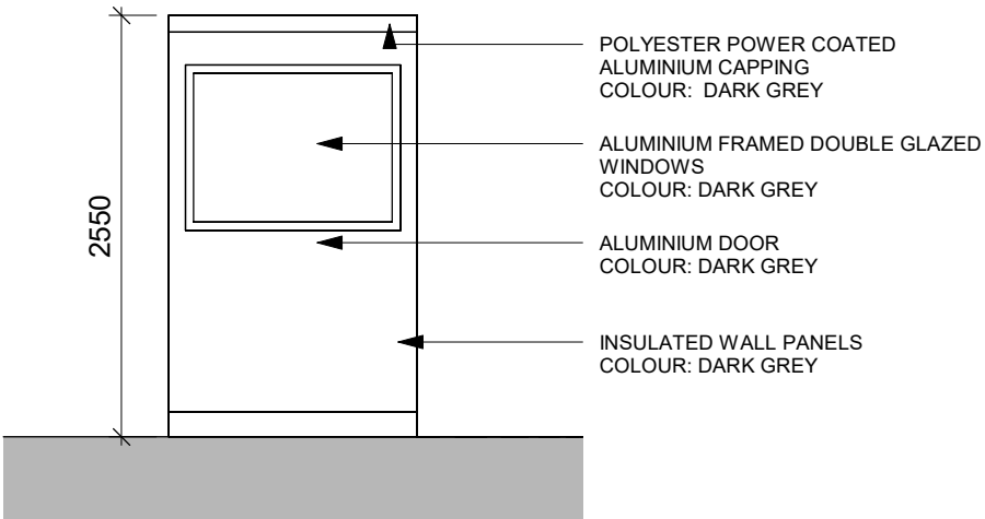
ELEVATION D 1:50
