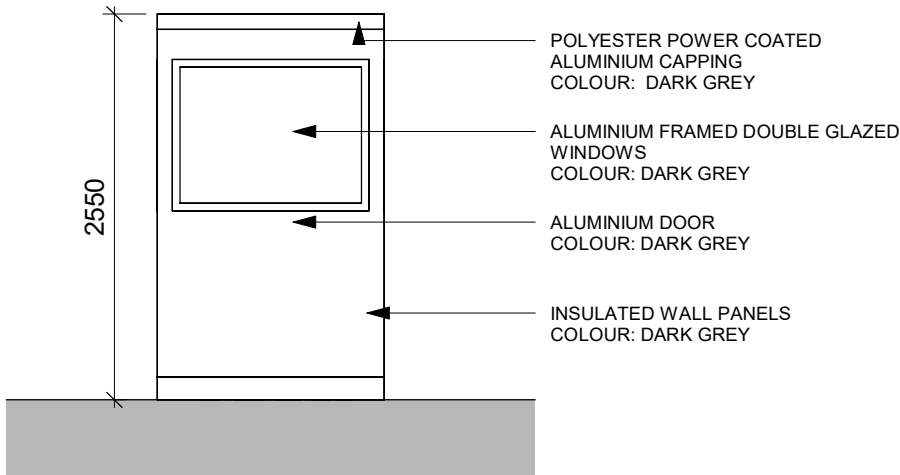
ELEVATION C 1:50
