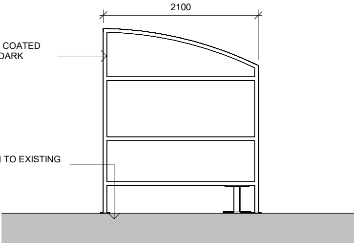
ELEVATION D 1 : 50
