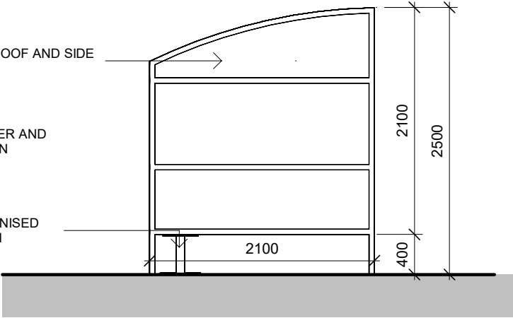
ELEVATION B 1 : 50
