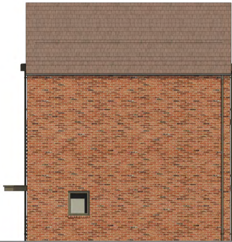
Right Elevation 1 : 100
