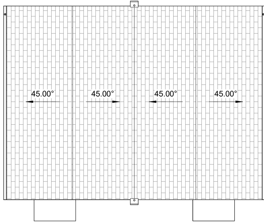
Roof Plan 1 : 100
