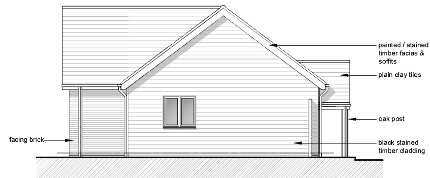
Flank Elevation
