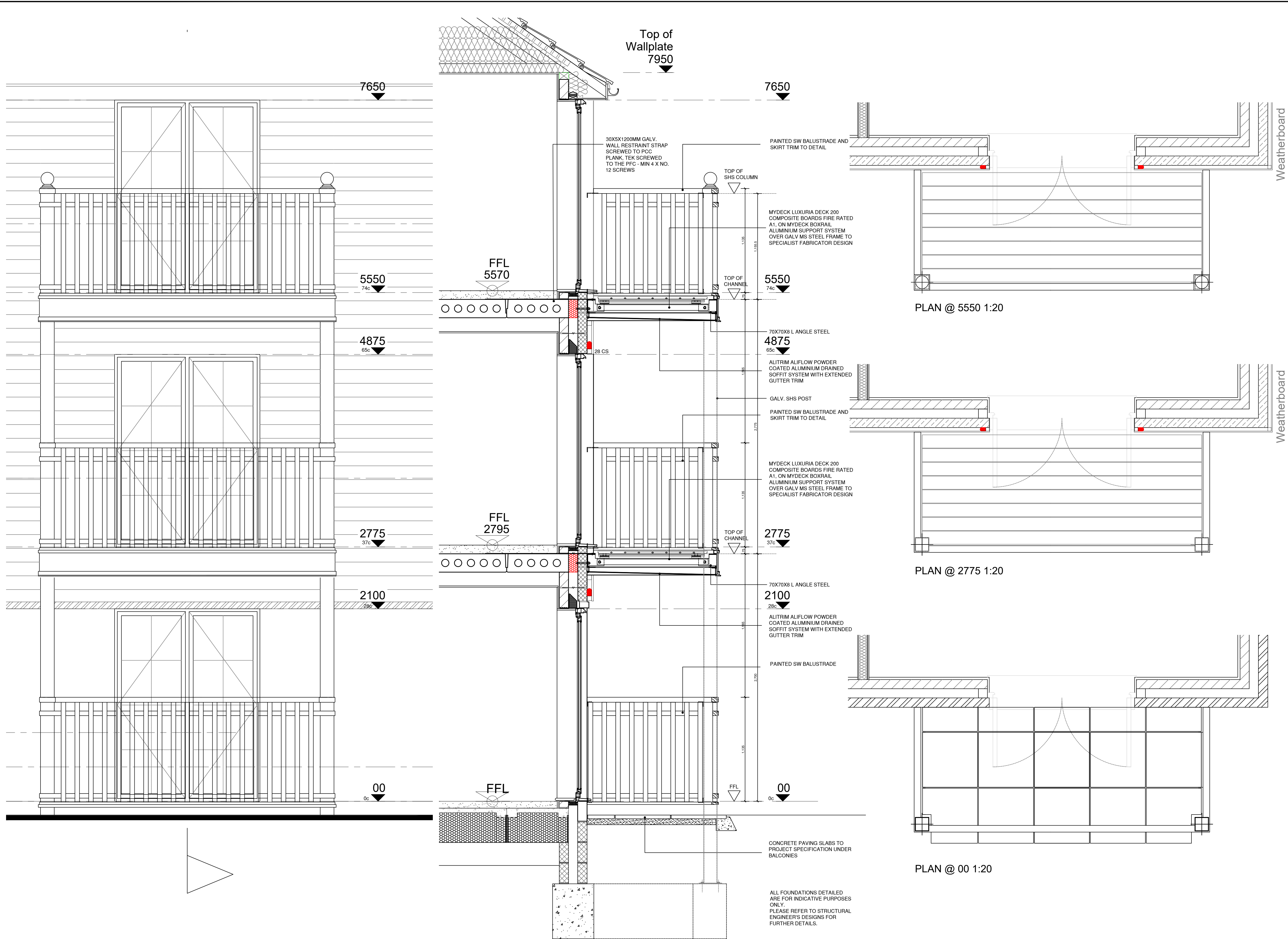
ELEVATION 1:20
