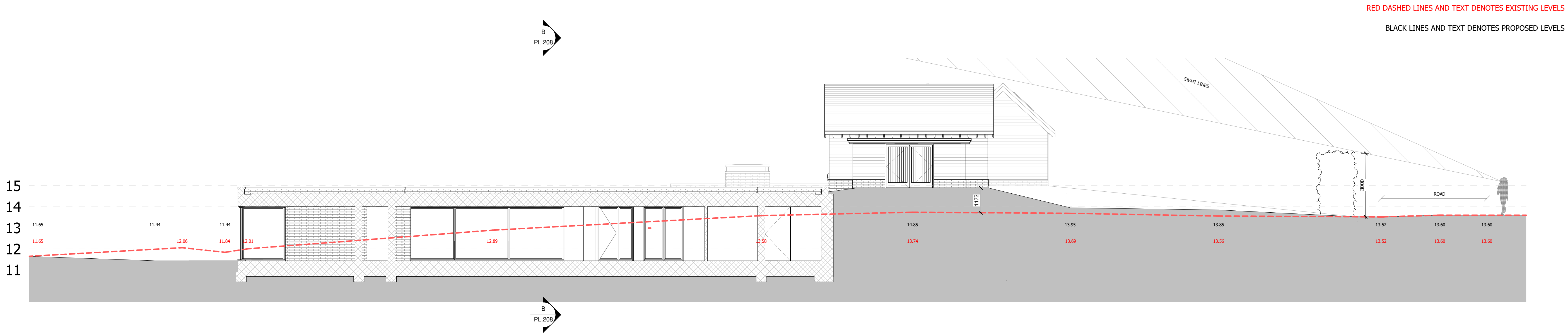
Site Section A-A - East - West 1 : 100
