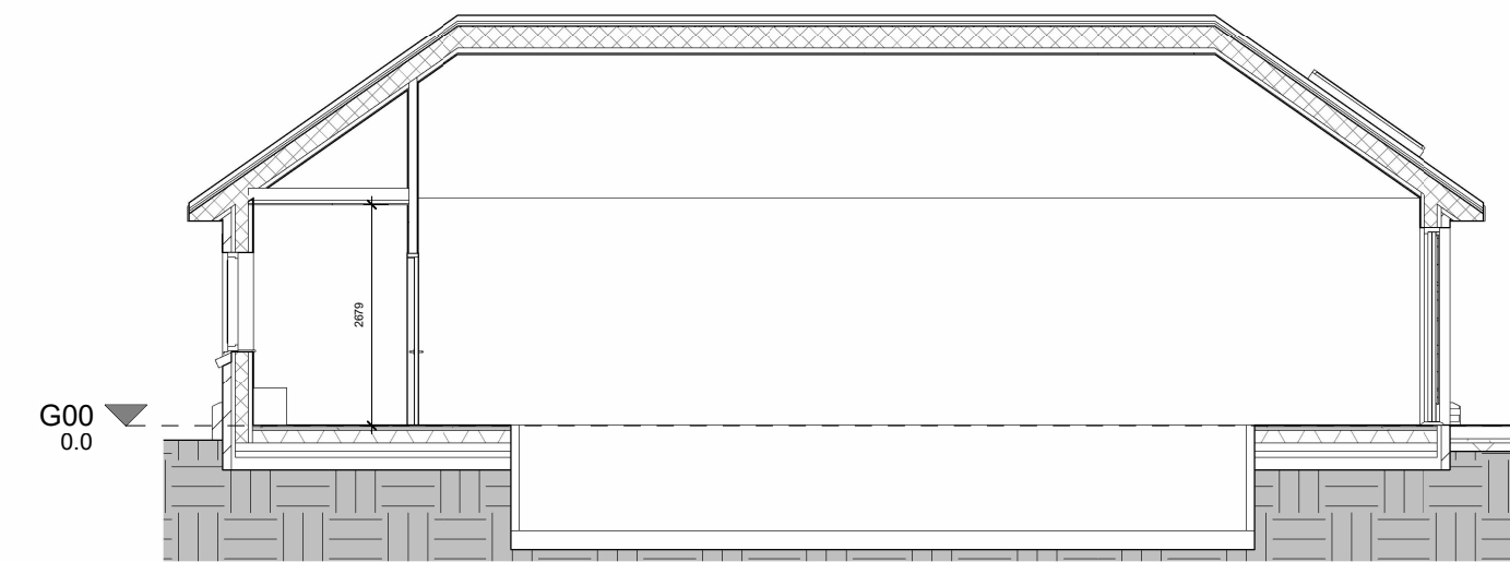
CC Section CC 1 : 100
