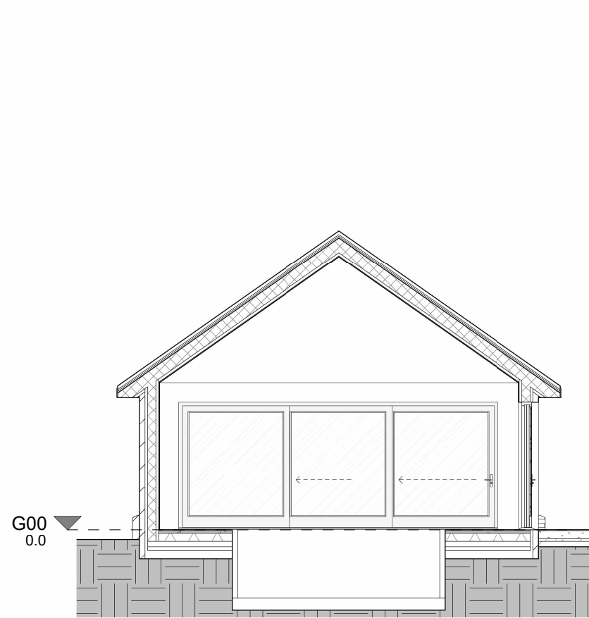
AA Outline Section AA 1 : 100
