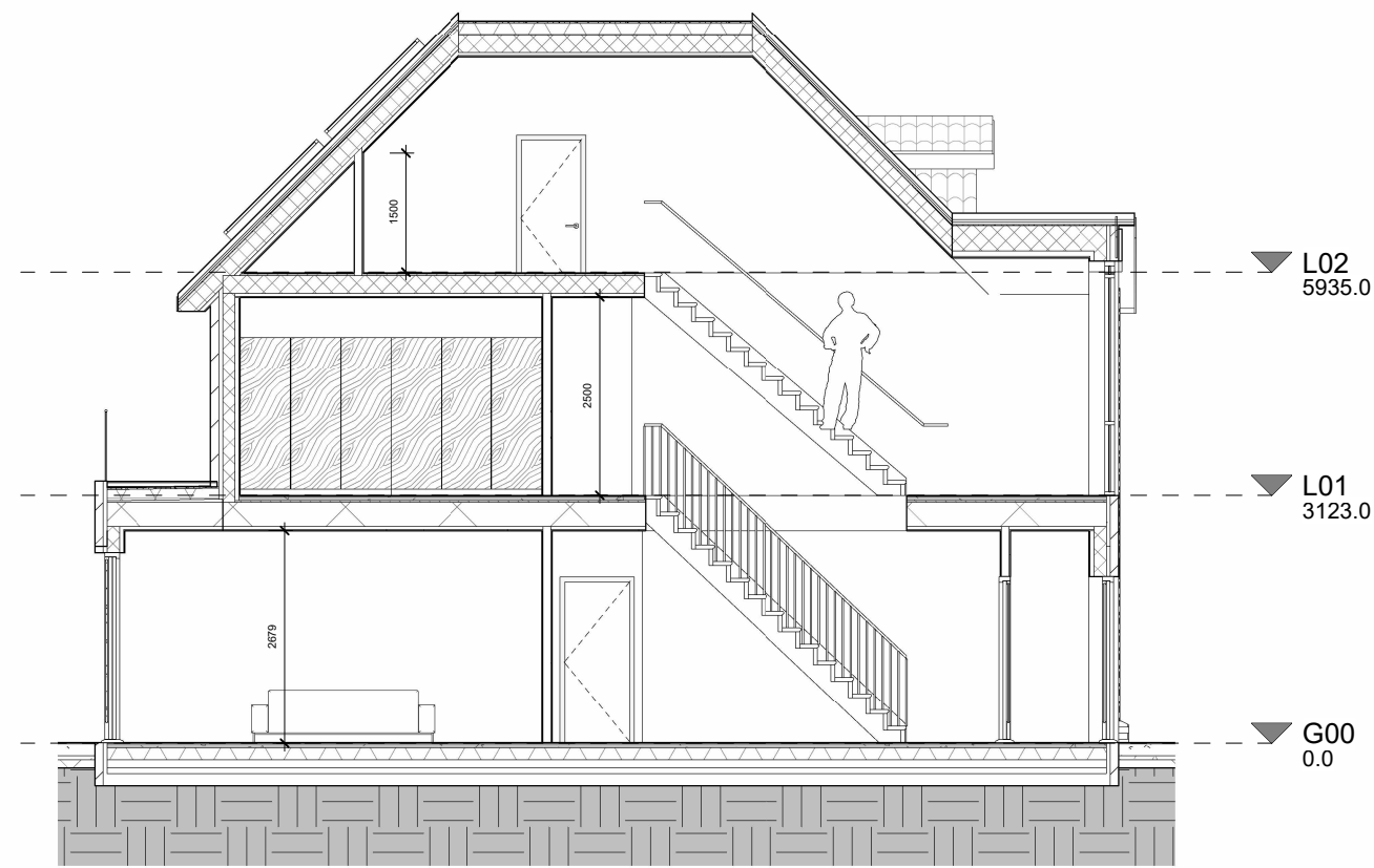
DD Section DD 1 : 100
