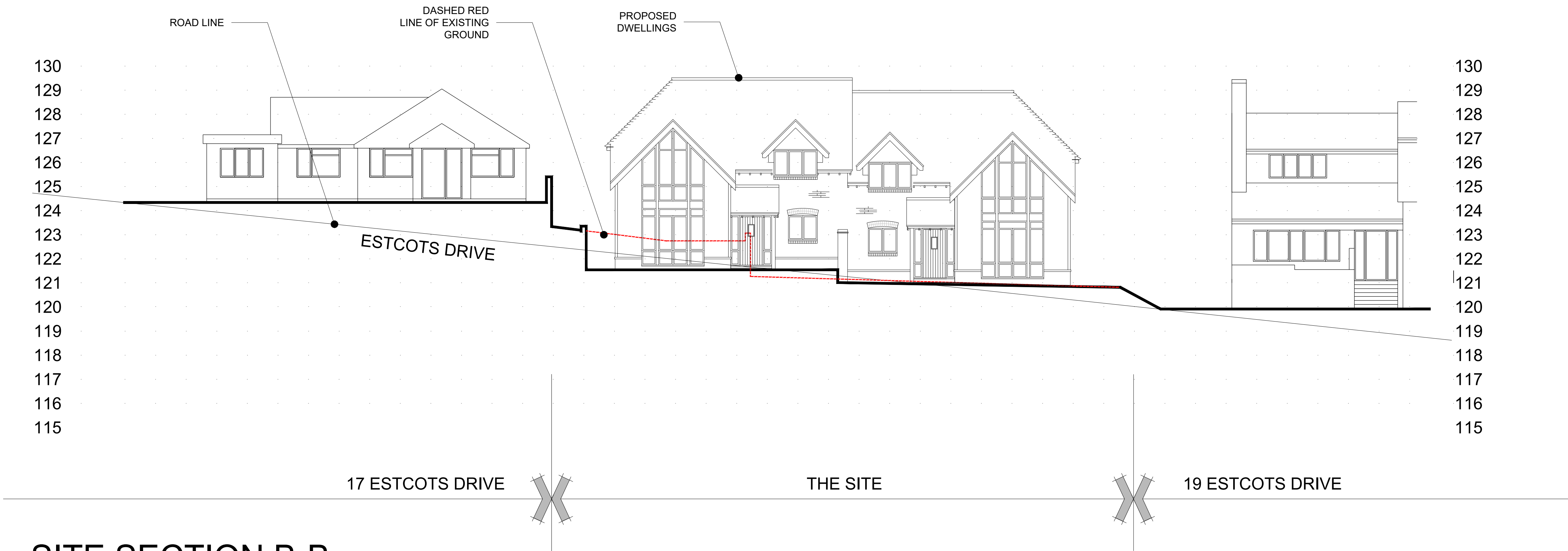
SITE SECTION B-B
