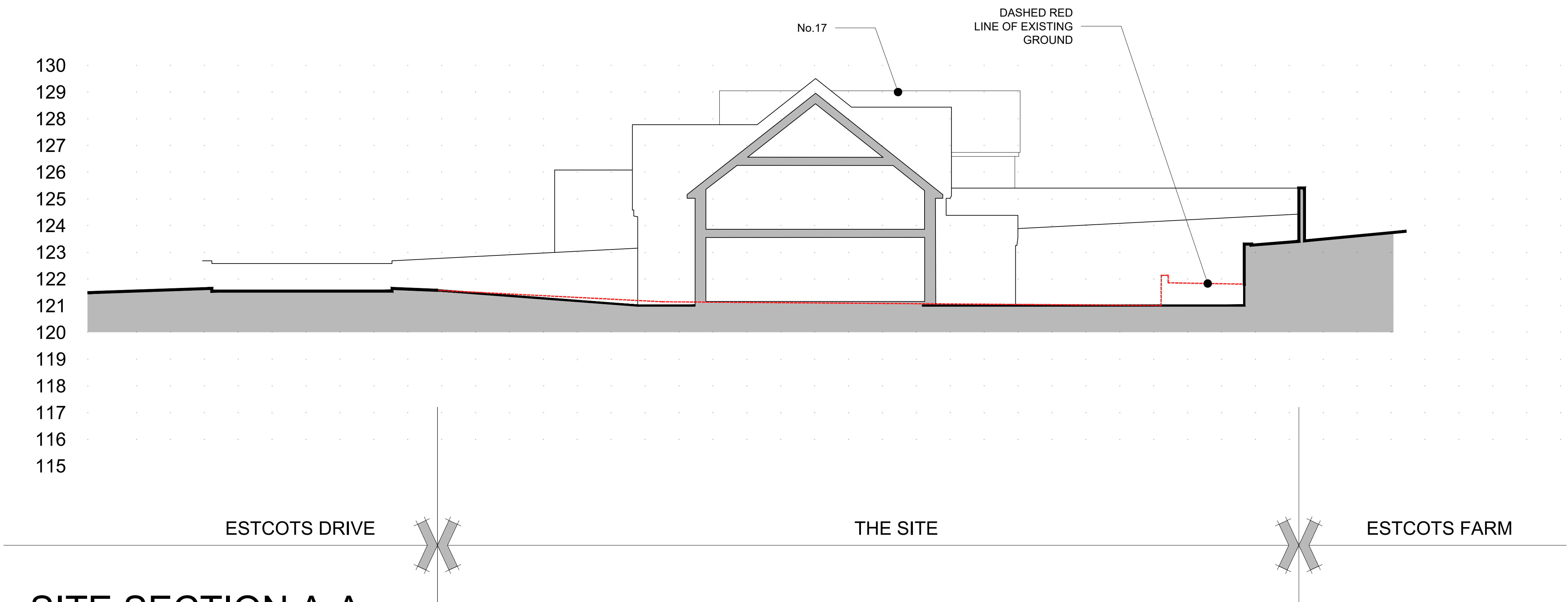
SITE SECTION A-A
