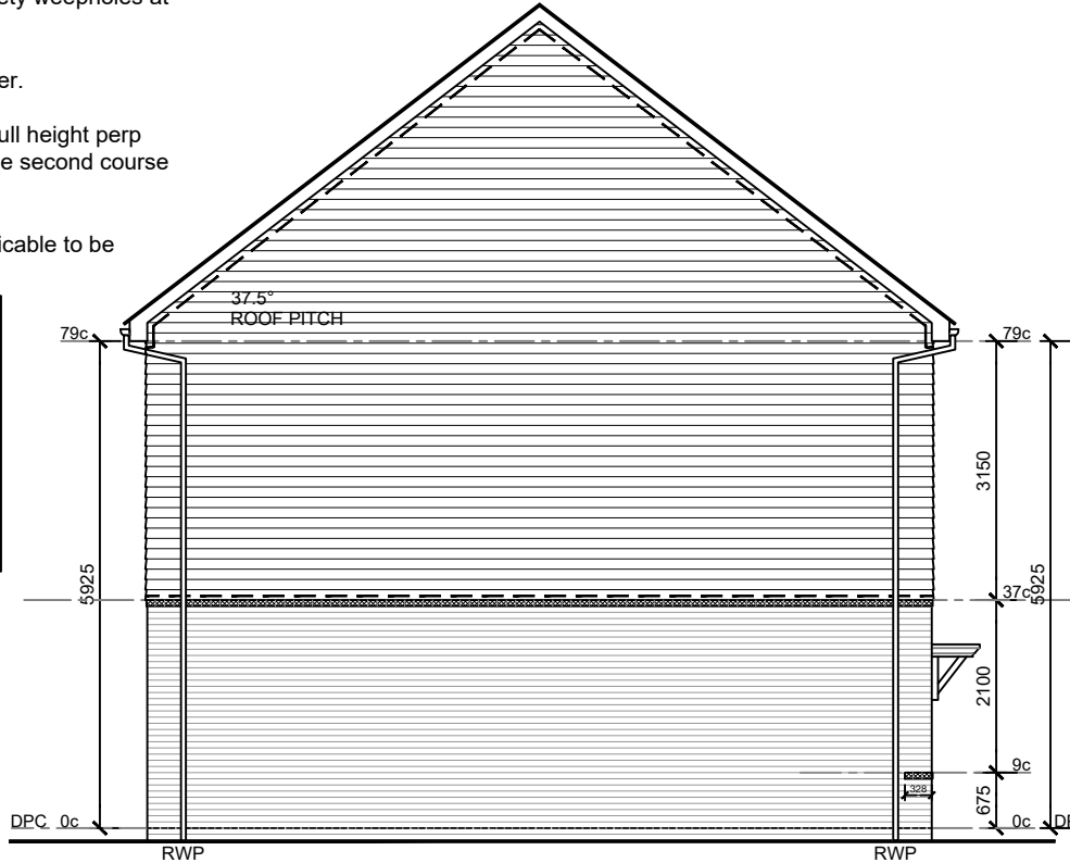
END ELEVATION
