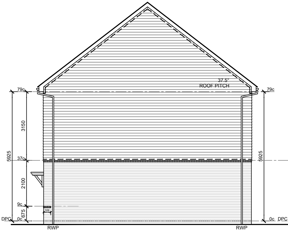
END ELEVATION
