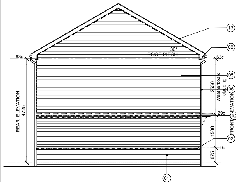
END ELEVATION
