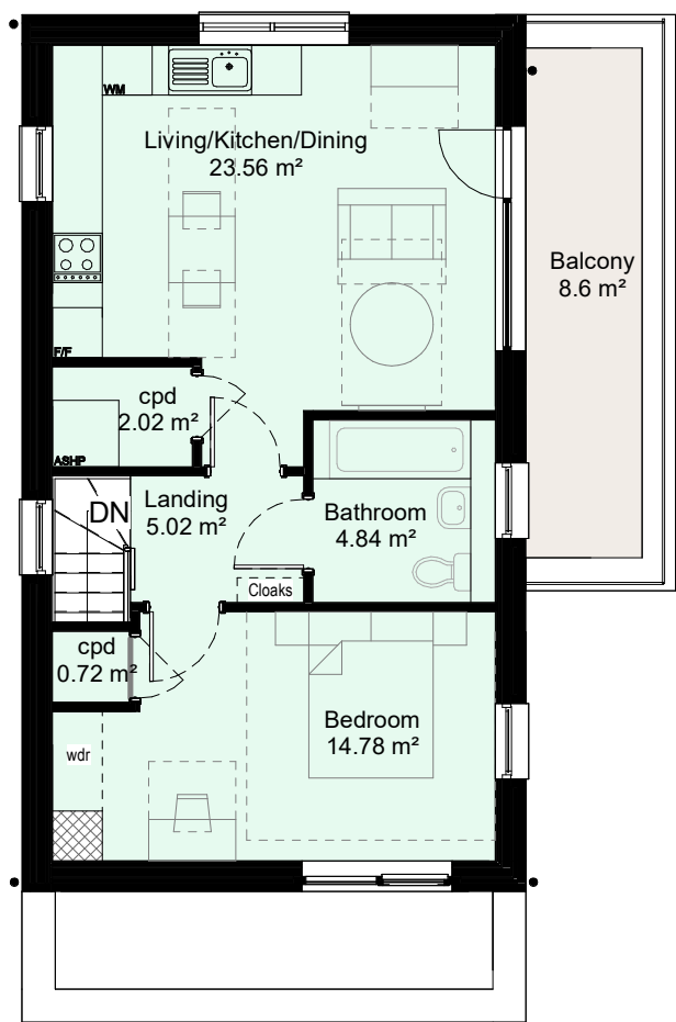
01 First FFL 1 : 100
