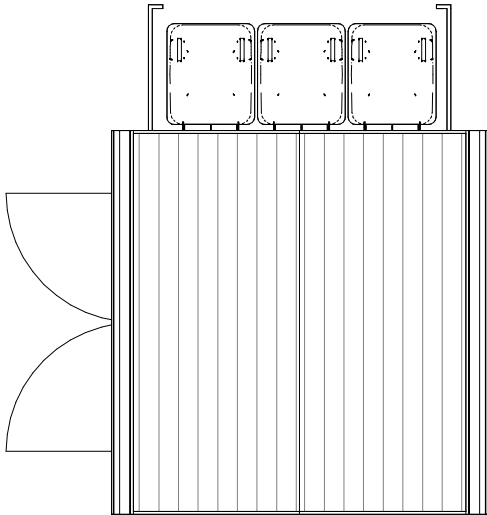
Roof Plan 1 : 50
