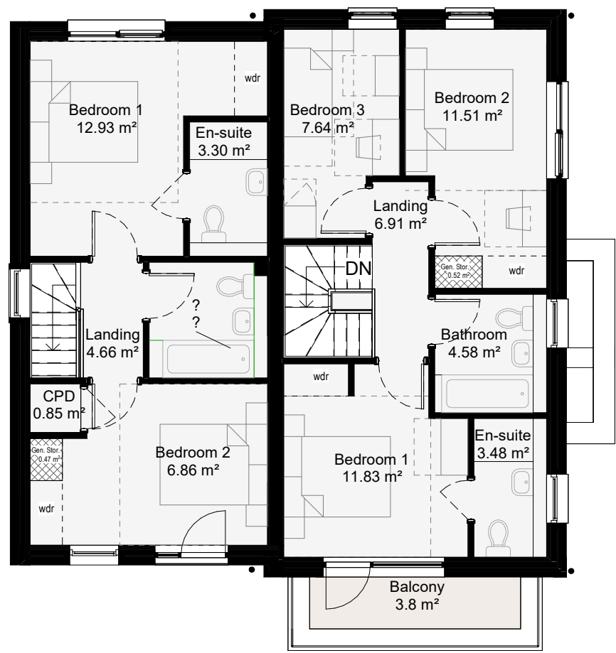
01 First FFL 1 : 100
