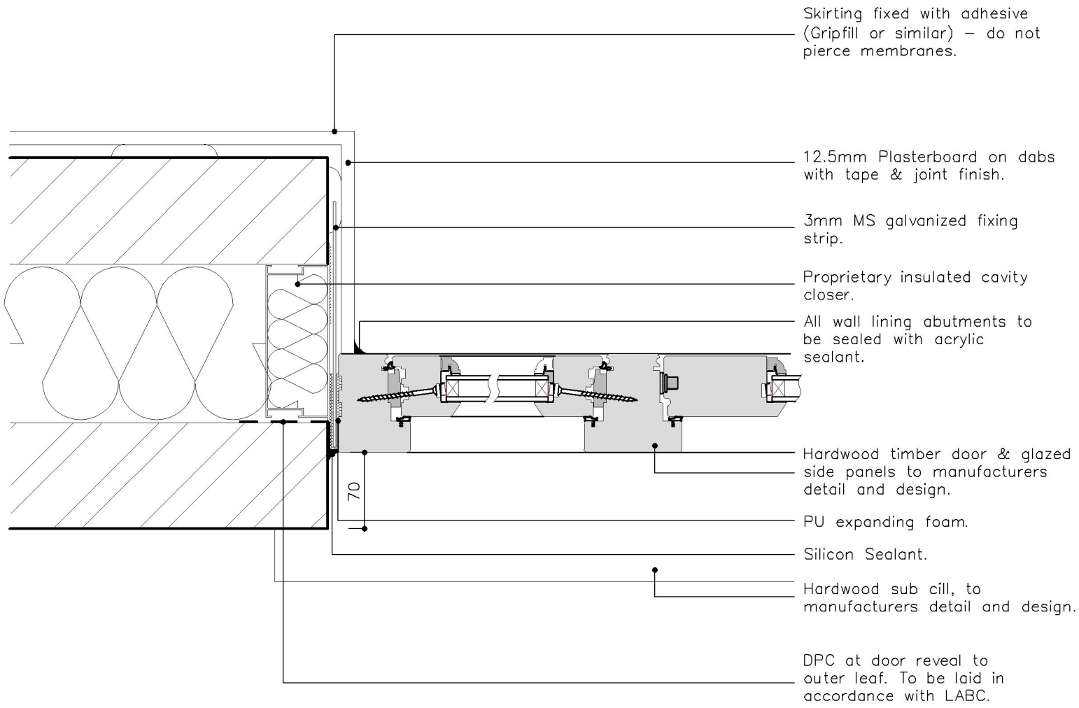
TIMBER DOOR JAMB DETAIL
