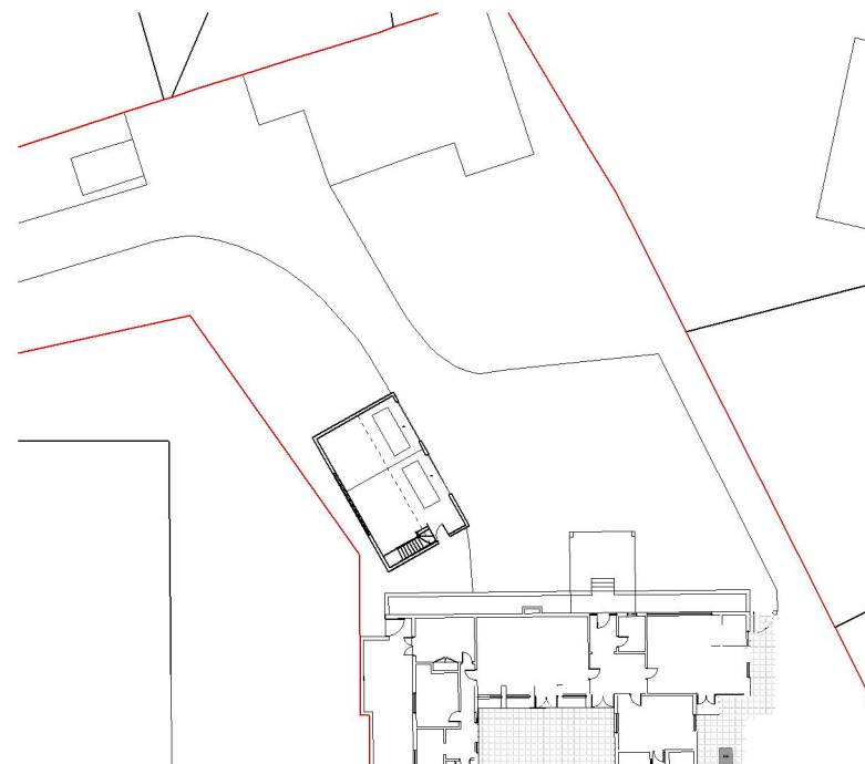
Site Plan 1:200
