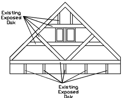
Existing Elevation 5
