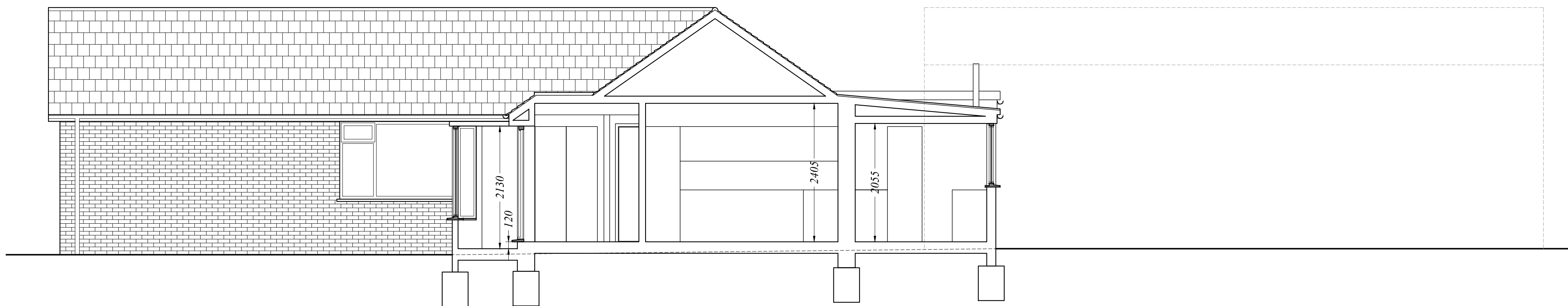
Section A-A
