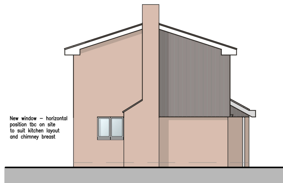
side elevation (sw) 1:100
