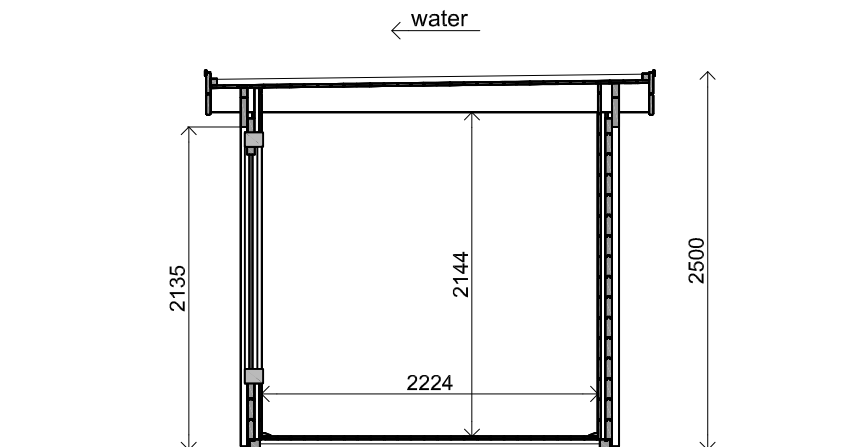
Doorsnede / Section / Durchschnitt 1-1
