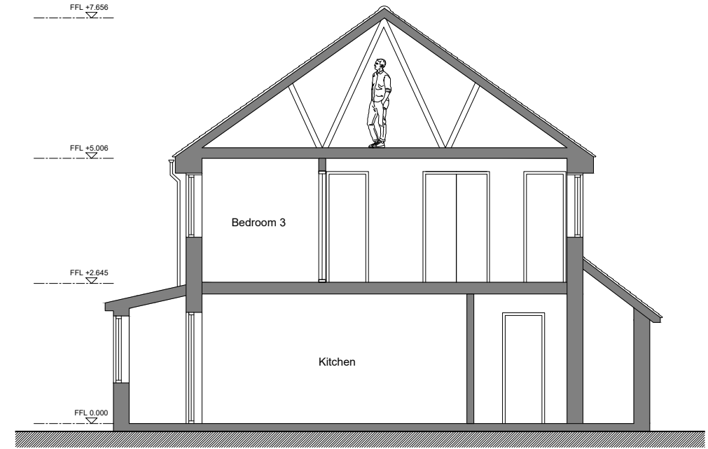
Existing Site Section 1:100
