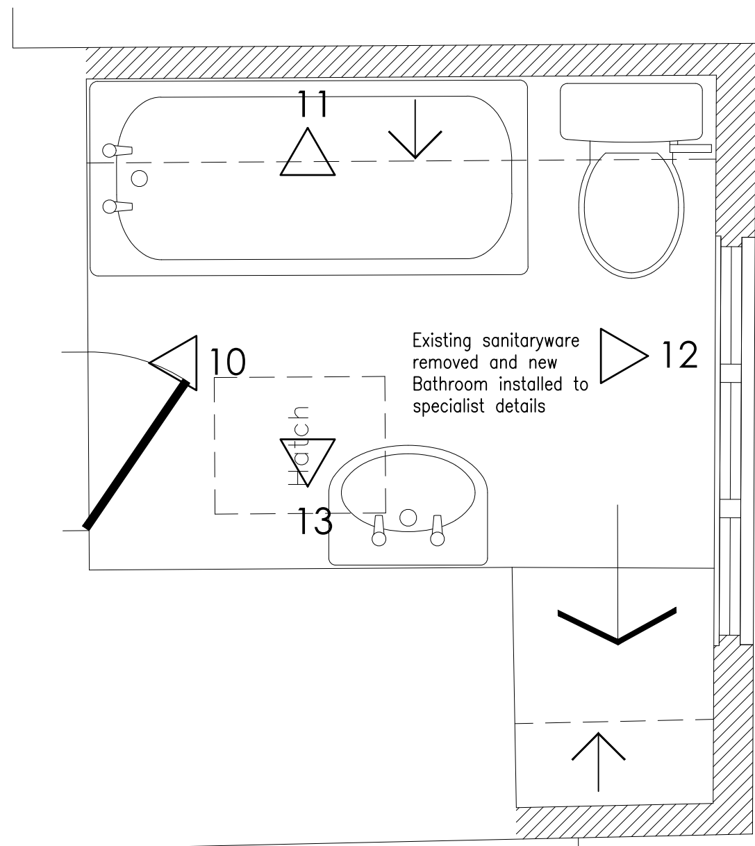
Plan 1:20
