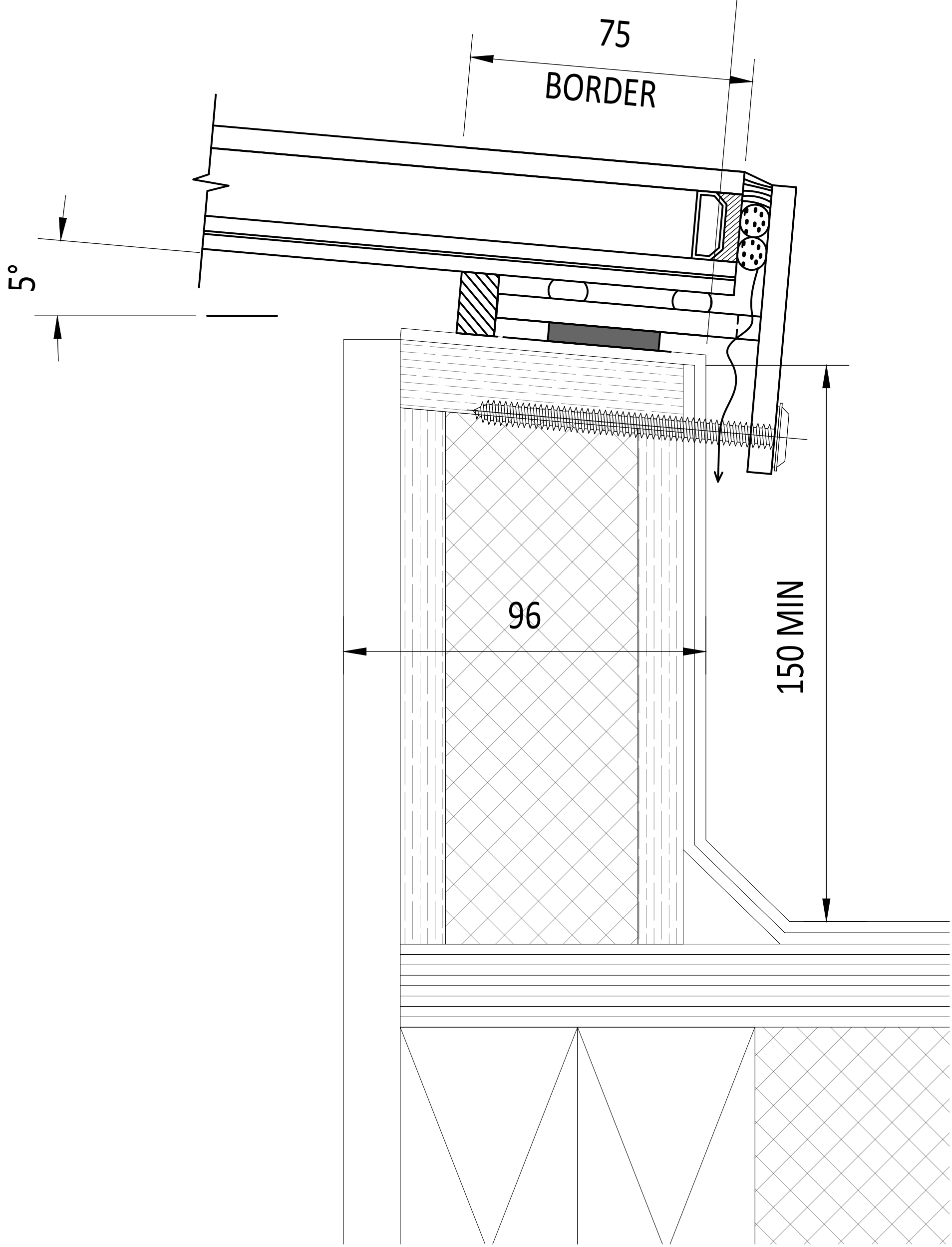
SECTION A-A
