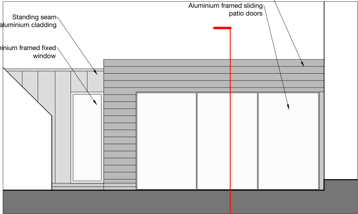
Elevation - 1:50
