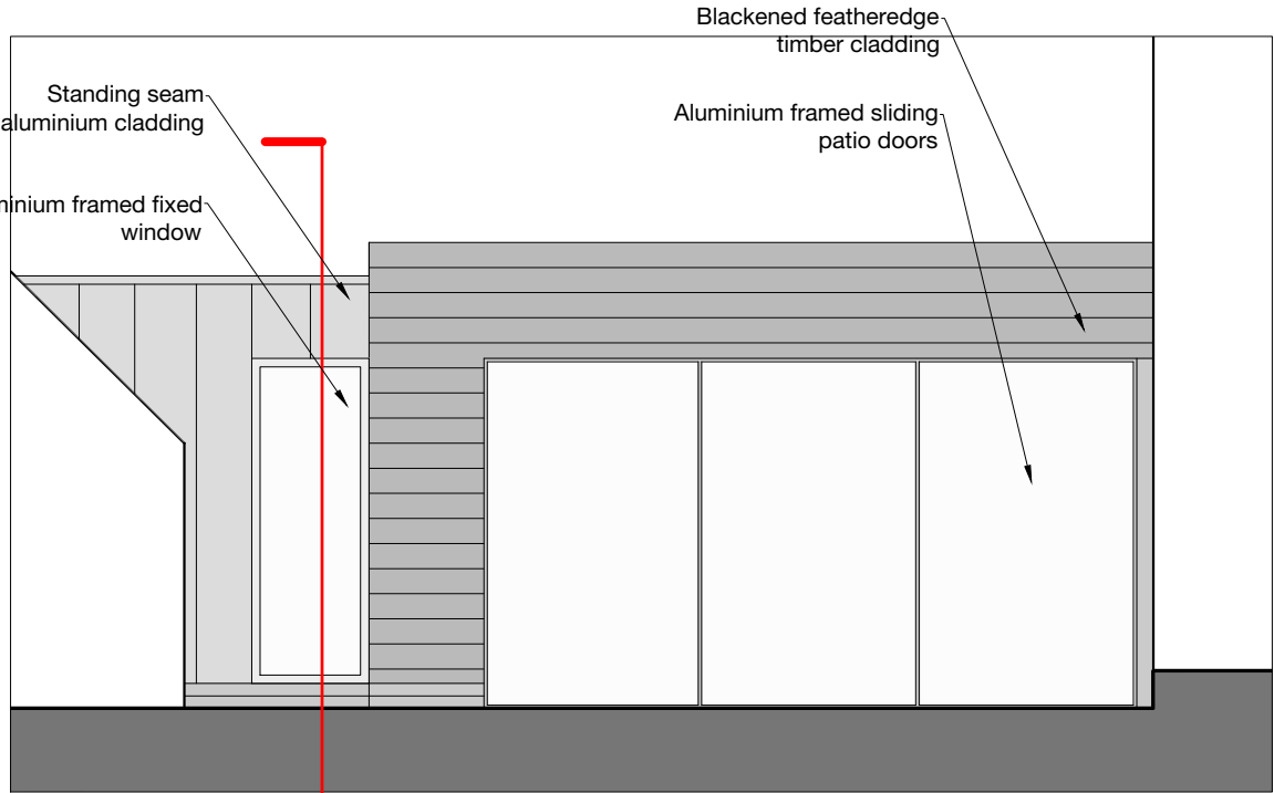
Elevation - 1:50
