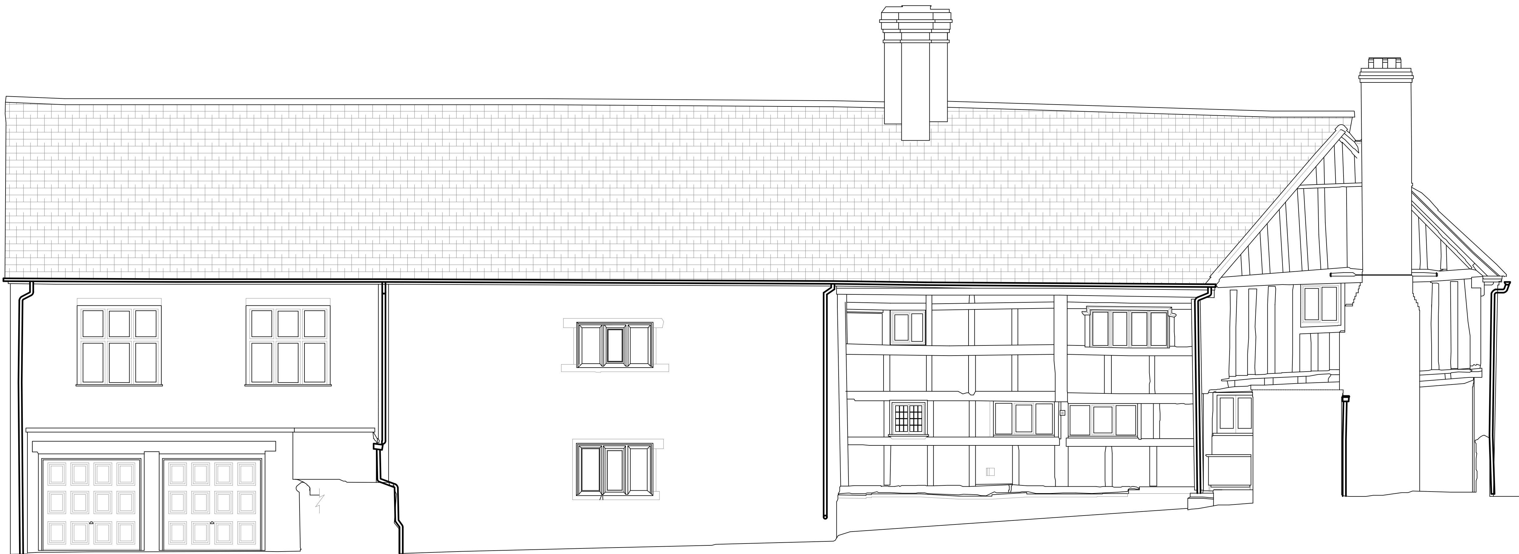
Datum: 51.00m. Elevation 2a.
