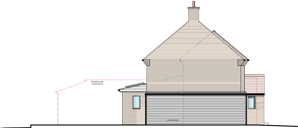
ELEVATION 4
