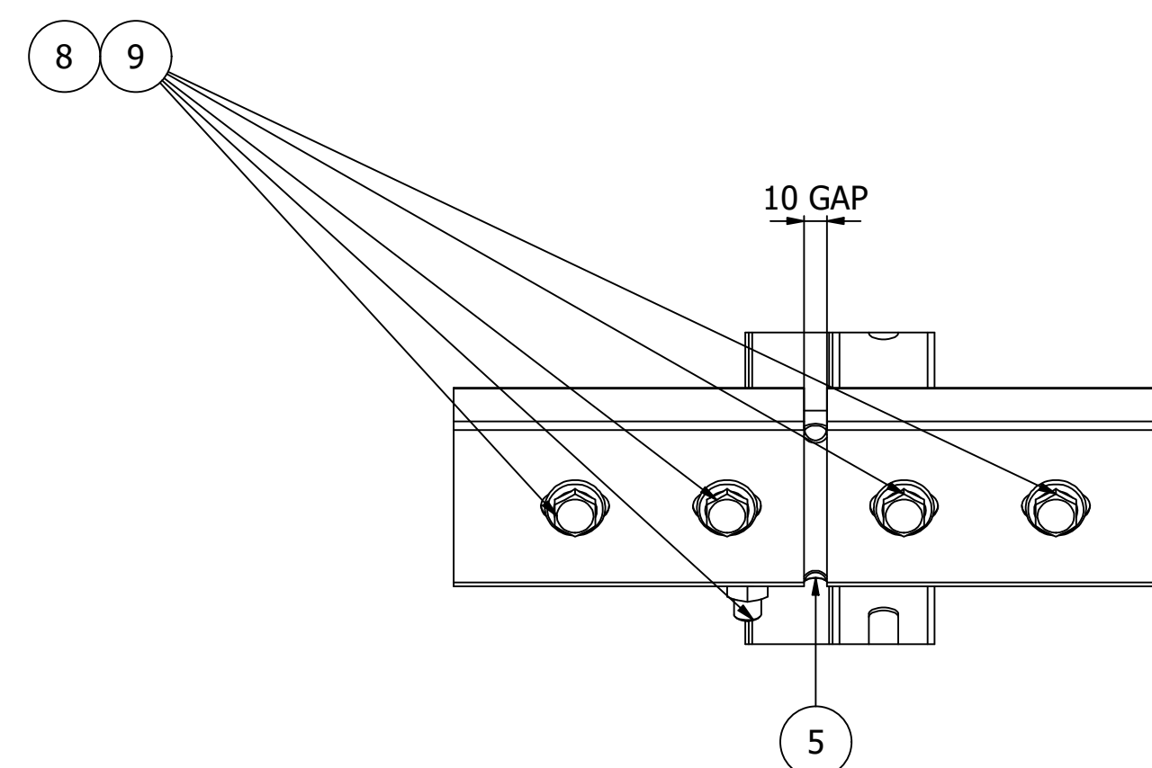
DETAILED VIEW A ( 1 : 3 ) TYP ALL POSNS
